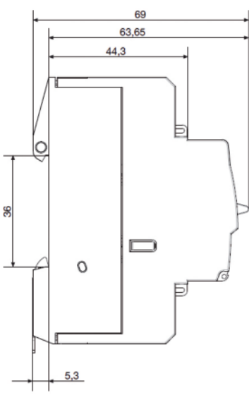
Zijaanzicht (met autoreset)
