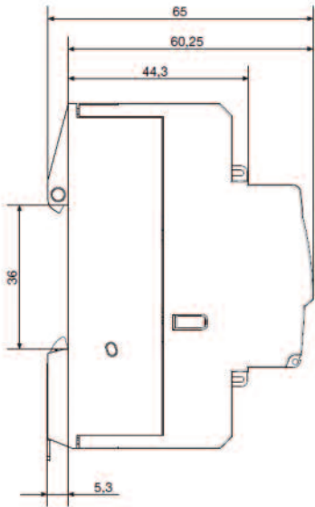
Zijaanzicht (handbediening)
