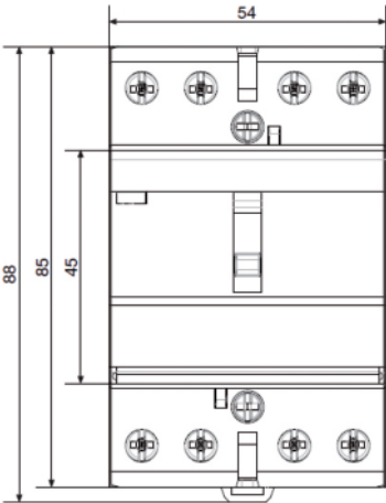
Vooraanzicht
