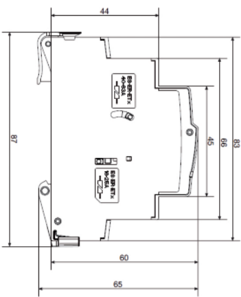
Zijaanzicht
